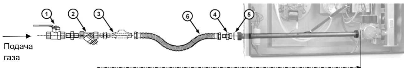
Рисунок 11.1 Подключение газа
