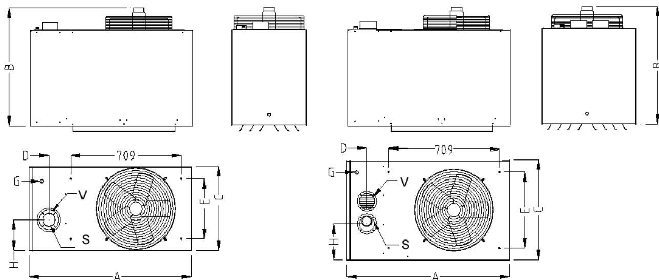
Рисунок 3.2.2 Внешний вид воздухонагревателя SA DT
