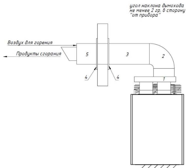
Рисунок 9.1.16 Горизонтальный коаксиальный дымоход SA1 0040/0050/0065/0085 DT
