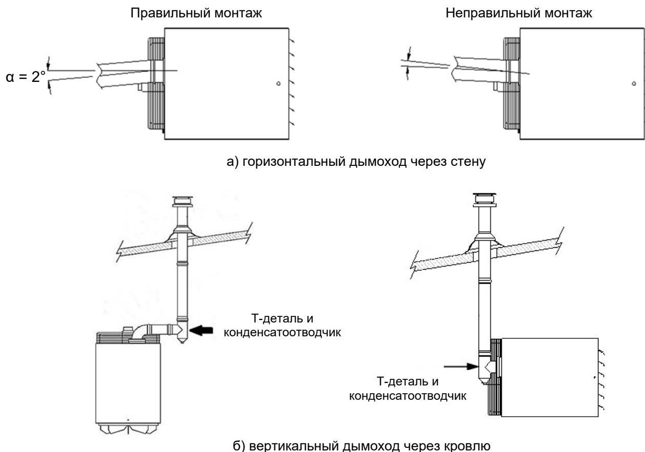
Рисунок 9.1.1 Монтаж дымоходов
