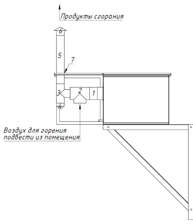
Рисунок 9.1.18 Стандартный комплект дымохода SA1 0020/0025/0030 RN
