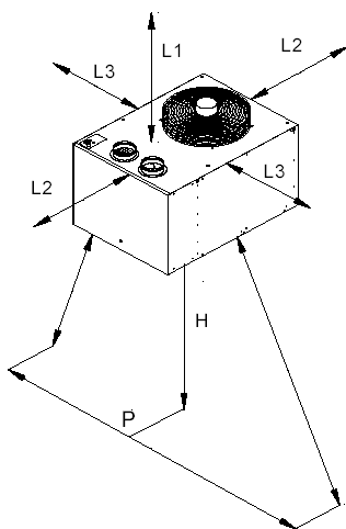
Рисунок 7.3.1 Монтажные расстояния воздухонагревателей- дестратификаторов SA1 DT
