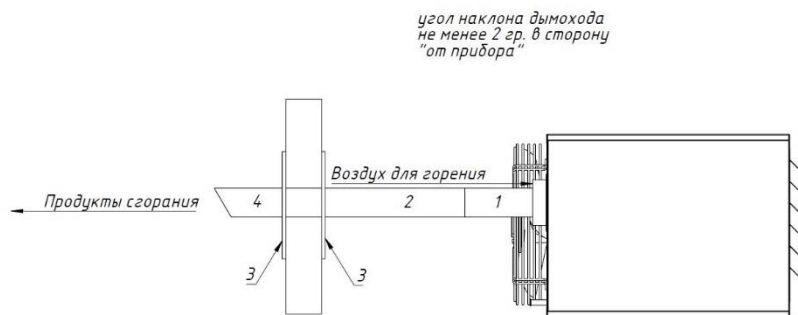
Рисунок 9.1.5 Горизонтальный одностенный дымоход SA1 0015/0020/0025/0030 A, SA1 0020/0025/0030 R.
