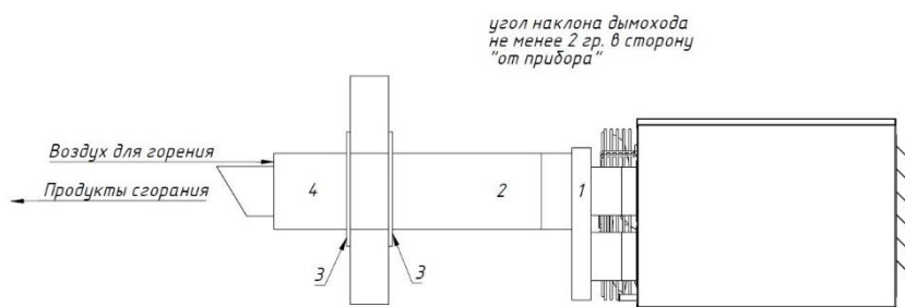
Рисунок 9.1.12 Горизонтальный коаксиальный дымоход SA1 0040/0050/0065/0085 A, SA1 0040/0050/0065/0085 R
