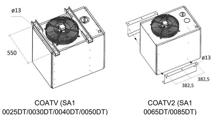
Рисунок 7.3.2 Комплект консолей
