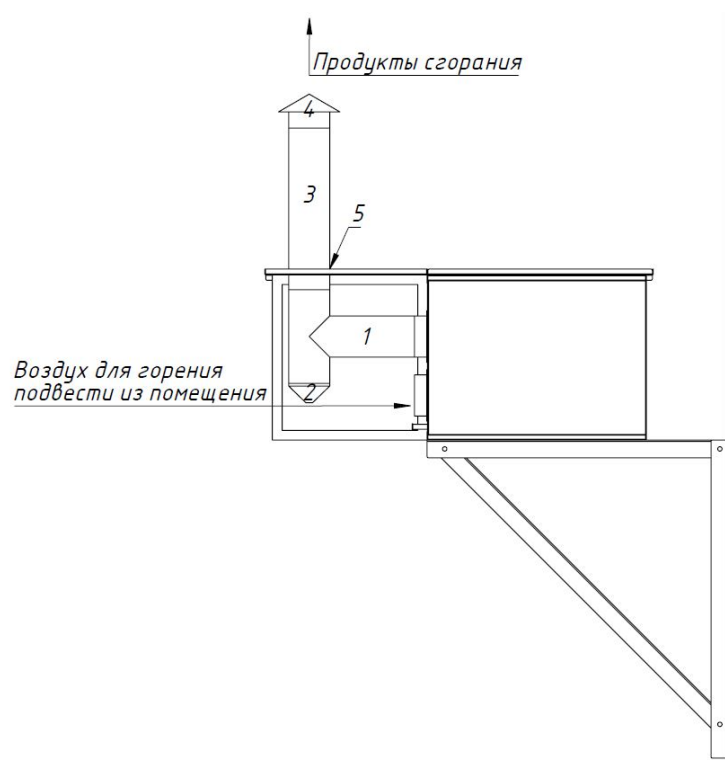
Рисунок 9.1.19 Стандартный комплект дымохода SA1 0040/0050/0065/0085 RN
