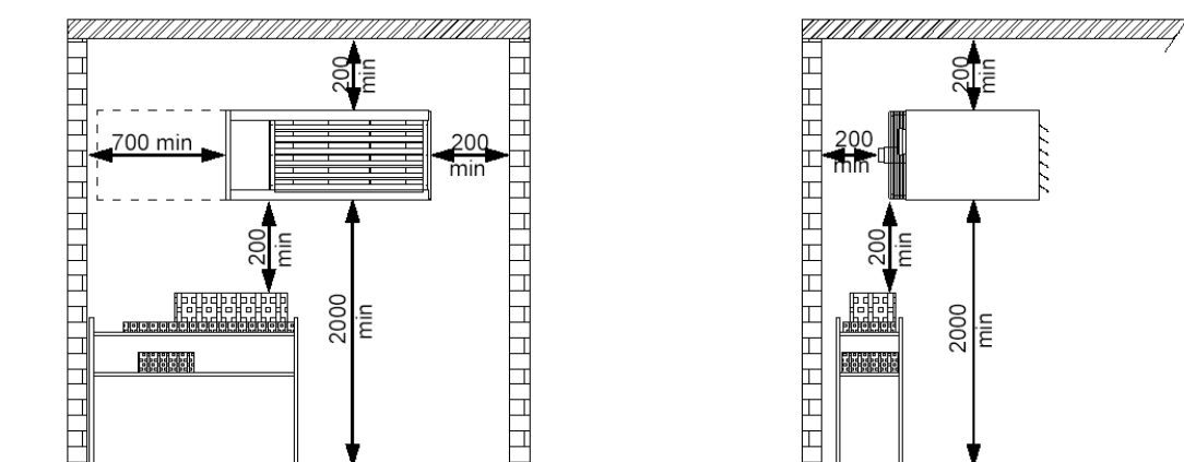
Рисунок 7.1.1 Безопасные расстояния от воздухонагревателя
