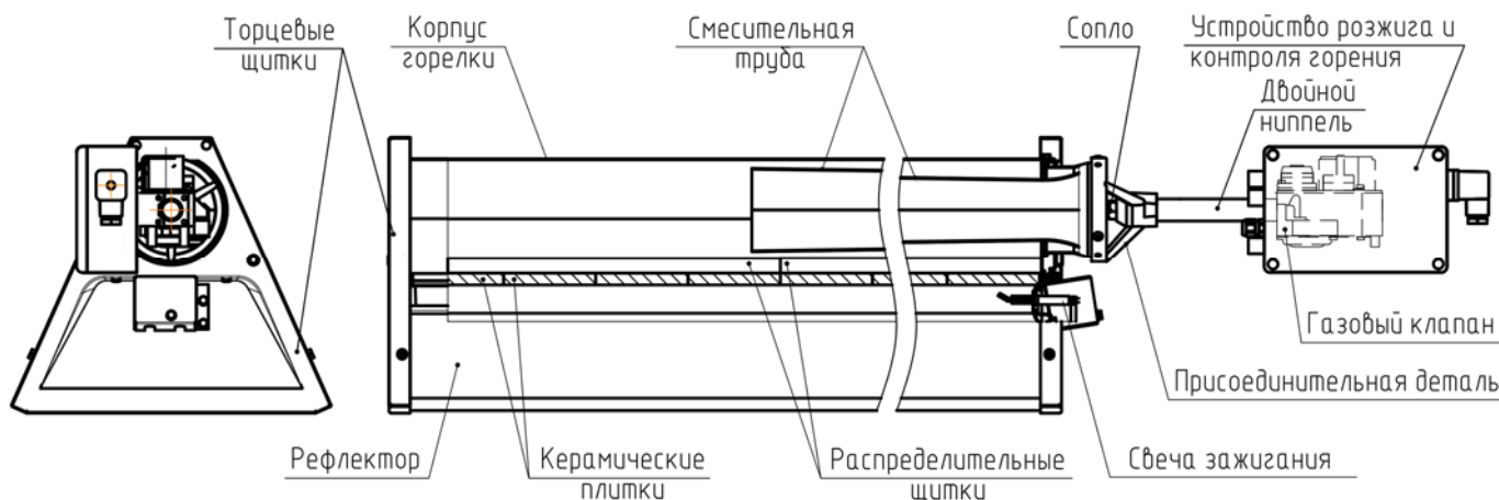
а) Излучатель с IC 3501
